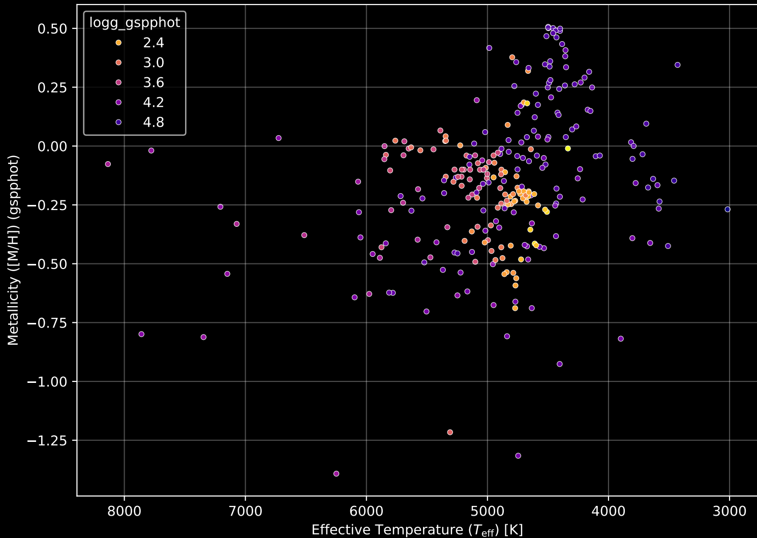
APOGEE DR17 Field: [178+36_btx] Stellar Population Parameters (n= 271)
